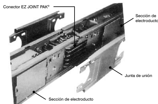
Sistema de unión del electroducto I-LINE II
